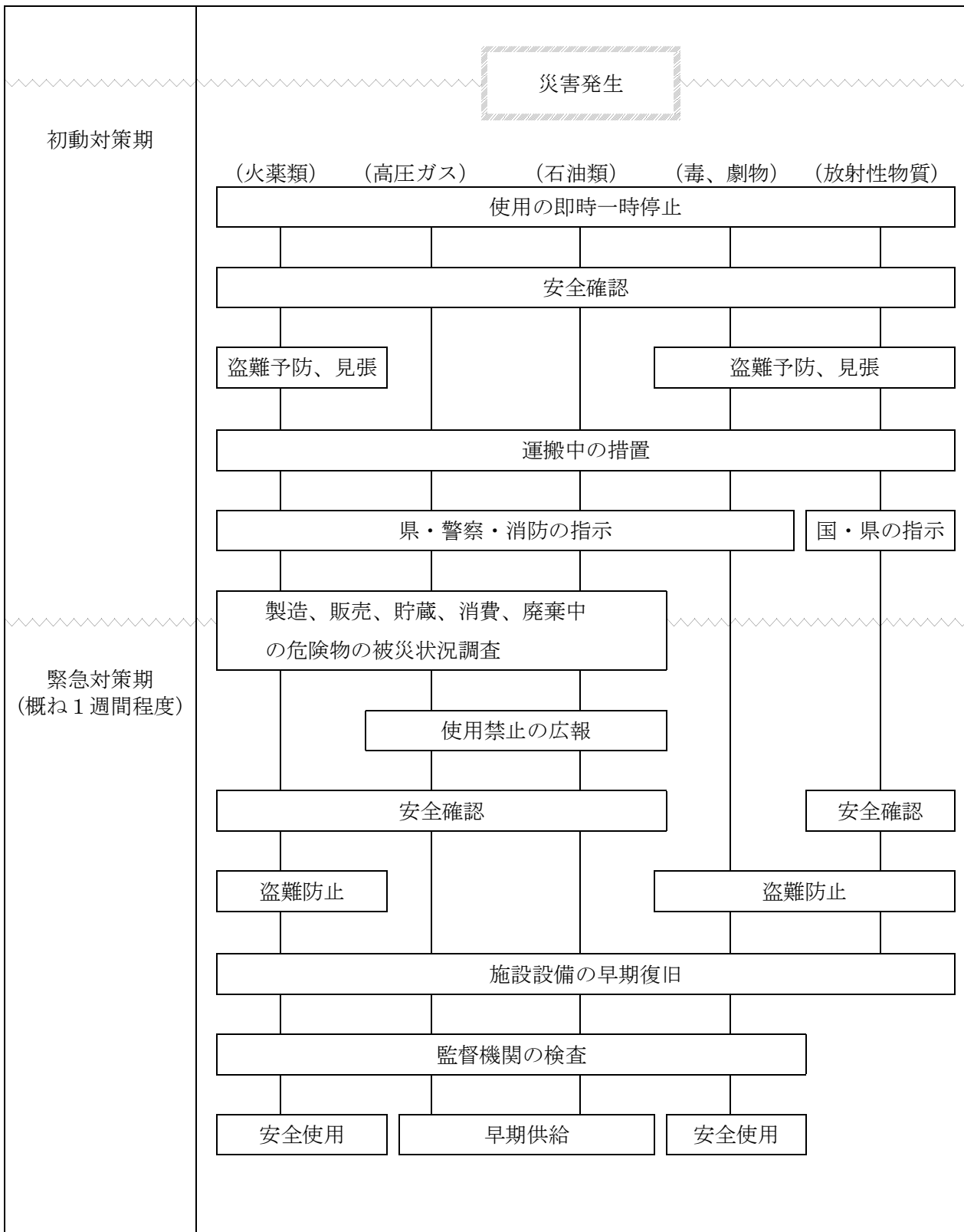
危険物の応急対策のフロー
